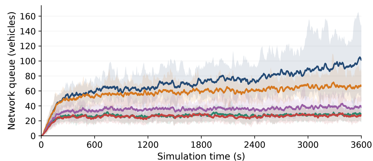
PPO
