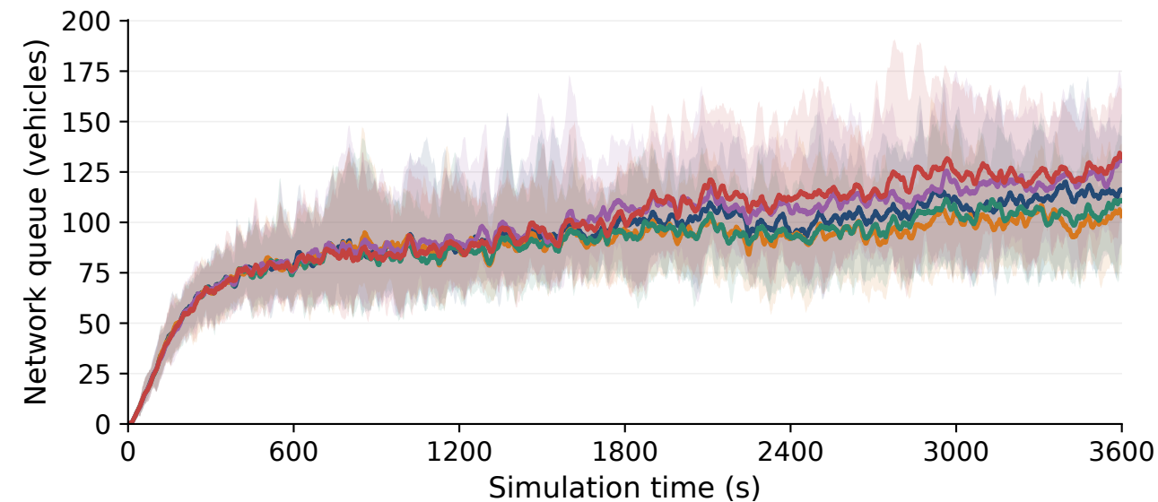
MA2C
